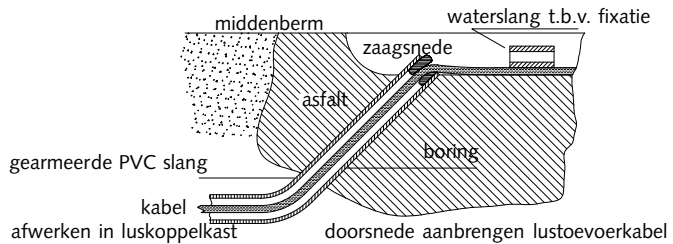
..... Figuur 5.9 Doorsnede aanbrengen lustoevoerkabel
