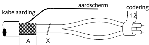
..... Figuur 5.12 Afwerking kabel voor luskoppelkast
