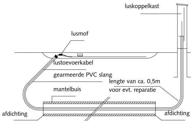
..... Figuur 5.10 Aanbrengen van lustoevoerkabel in mantelbuizen
