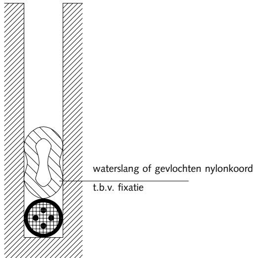
..... Figuur 5.8 Fixeren van lustoe- voer- en luskabel in zaagsnede
