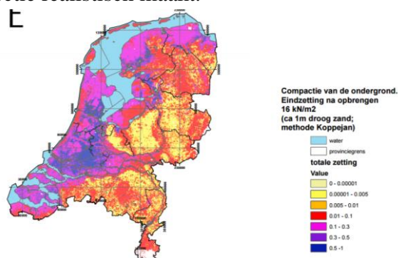
Figuur 4. De zettingsgevoeligheid van de Nederlandse ondergrond (7).
