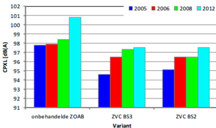
Figuur 2: CPX-niveaus op de A15 gemeten in 2005, 2006, 2008 en 2012 bij 80 km/u.
