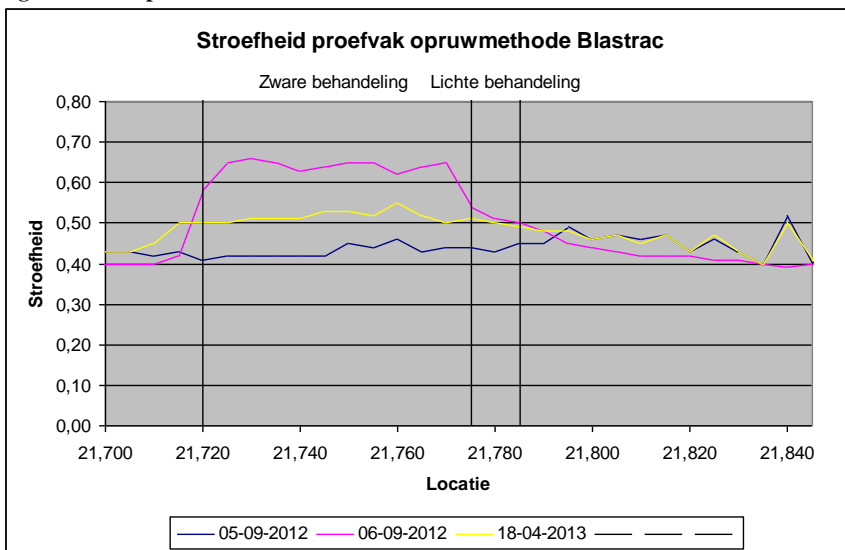
Figuur 1 Verloop van de stroefheid
